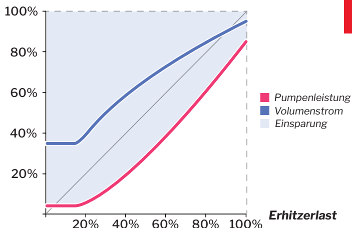
Pumpenleistung / Volumenstrom
